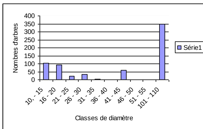
Fig 8. La distribution des arbres de dhp > 10cm des différentes espèces.
