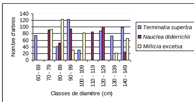
Figure 9. Structure diamétrique de Terminalia superba , Nauclea diderrichii et Millicia excelsa .
