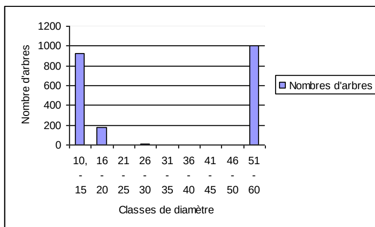
Fig 4. Distribution de nombre d'arbres (à dh \geq 10 cm) pour les différentes catégories de diamètre.
