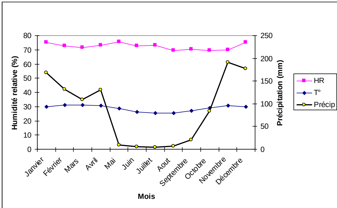
Figure n°1 : Diagramme ombrothermique moyenne de 2002 à 2005
