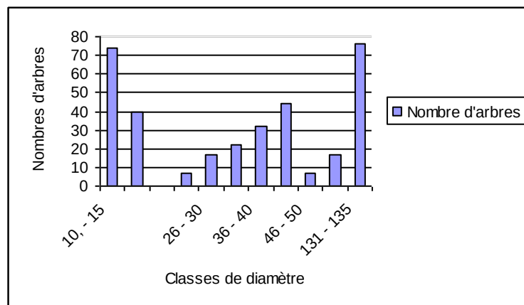
Fig 6. La distribution des arbres de dhp \geq 10cm des différentes espèces
