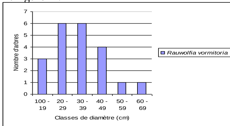
Figure 11. Structure diamétrique de Rauwolfia vomitoria .
