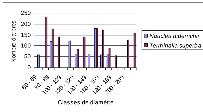
Figure 3. Structure diamétrique de Nauclea diderrichii et Terminalia superba
