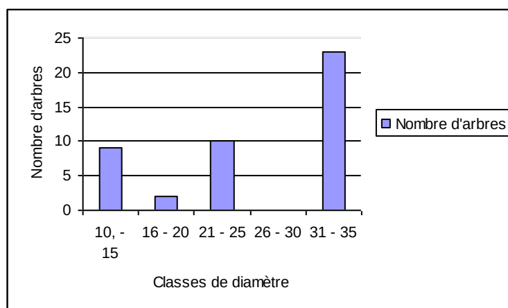
Figure 10. Distribution des arbres de dhp ≥ 10 cm des différentes espèces.
