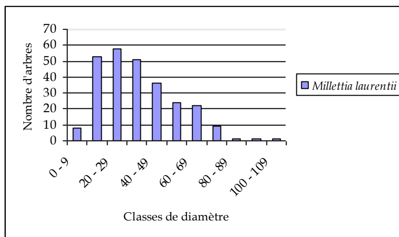
Fig 12. Structure diamétrique de Millettia laurentii
